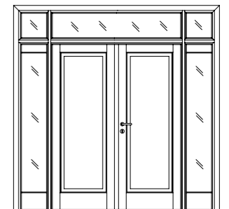
Doppio battente con fianchi-luce e sopraluce Double-leaf door with side-lights and transom
